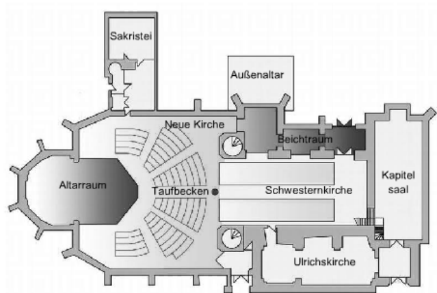
Oben: Pfarr- und Wallfahrtskirche Rulle: Grundriss heutige Aufteilung nach der jüngsten Renovierung und Neuordnung – Bildnachweis: Katholische Kirchengemeinde Rulle (vgl. im Internet: http://www.st-johannes-rulle.de/index.php/home/unsere-kirchen ; unten: Ansicht Innenraum, Blick von der „Neuen Kirche“ in die „Schwesternkirche“ – Bildnachweis: Norbert Linke, Rulle
